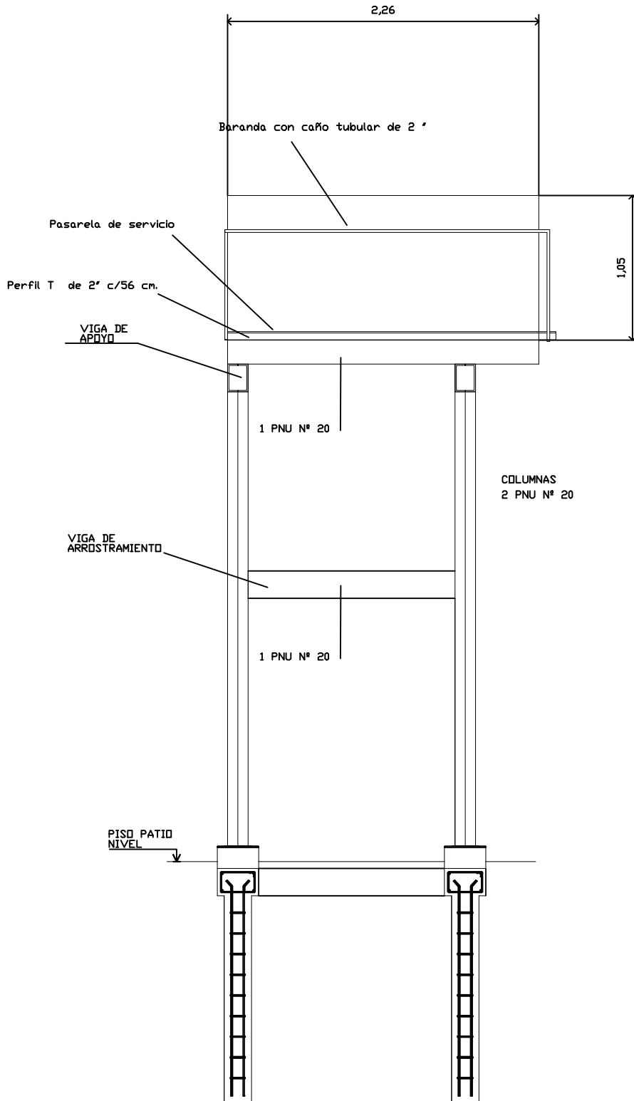
CORTE B-B
