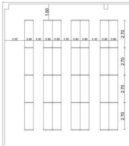
Armado en Planta de los 28 Módulos de 2.70m
